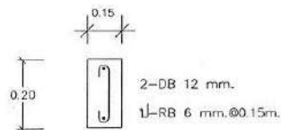
ด้าน B1
