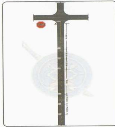
รูปที่ ๒๐ รูปแบบการติดตั้งชุดแถบชะลอความเร็วก่อนถึงจุดที่ต้องการเตือน
